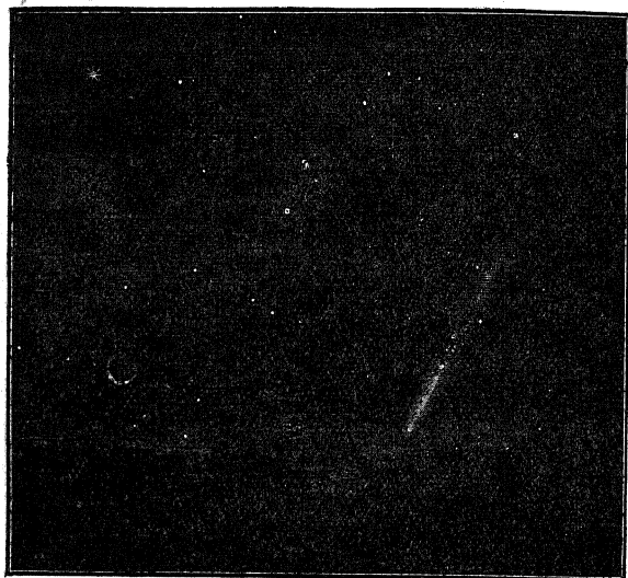
चित्र ८—सन् १८८२ का पुच्छलतारा
